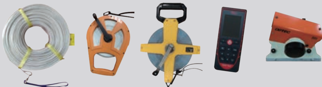
量距是地政測量最基本的工作，隨著時代進步，儀器也越來越精密。圖為從早期到現在所使用的各式量距工具，從左至右依序為測繩、皮捲尺、鋼捲尺，到精密度更高的手持式測距儀、平板光波測距儀。
