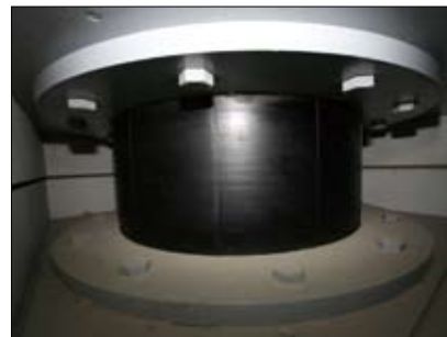
隔震層共使用36個隔震墊吸收地震震度。
